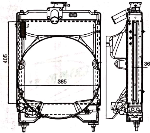
TAFE 1035 DI STUBNOSE CORE - B-8124242029ALU
