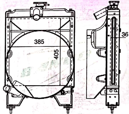
TAFE 1035 DI (J) MAHASHAKTI RADIATOR - B-8124252080ALU, CORE - B-8124252029ALU
