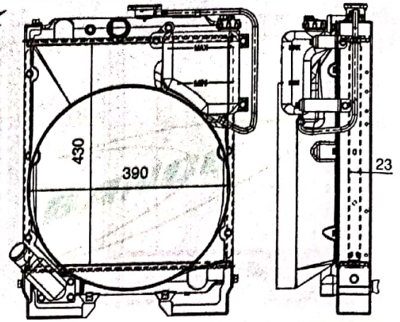
TAFE 25 DI RADIATOR Core - 8124232029ALU
