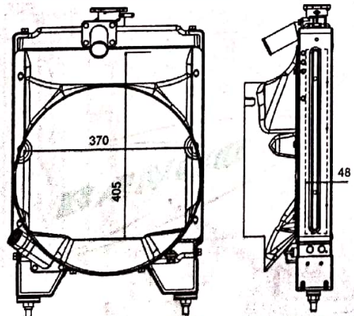
TAFE 241 EAGLE / 245 DI (J) 45 HP (MAHASHAKTI) RADIATOR - 8124262080ALU CORE - B-8124262029ALU
